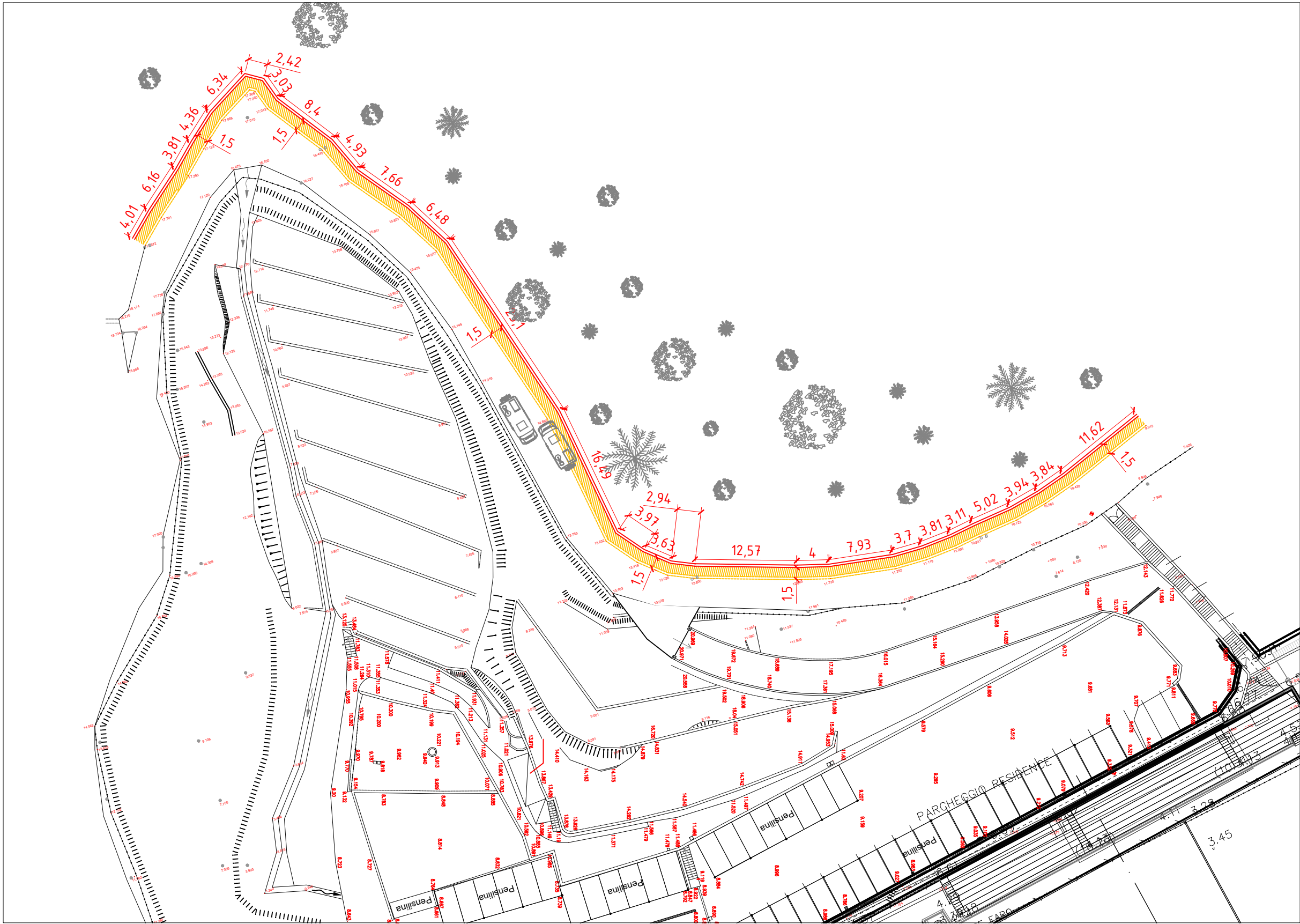
Planimetria - scala 1500
